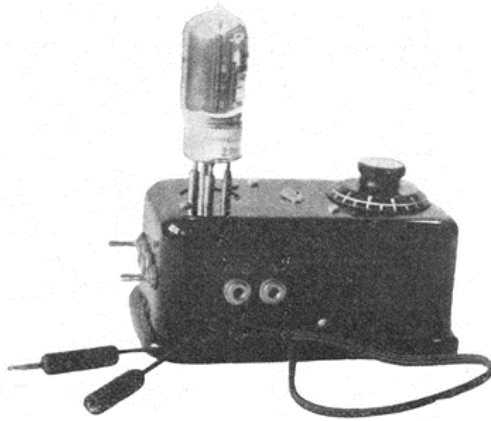
1 lampas lēnmaiņas pastiprinātājs
