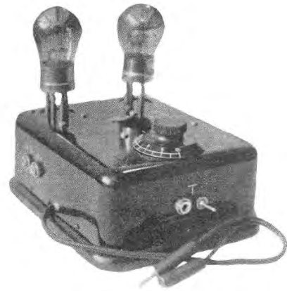
2 lampiņu zemperioda pastiprinātājs
