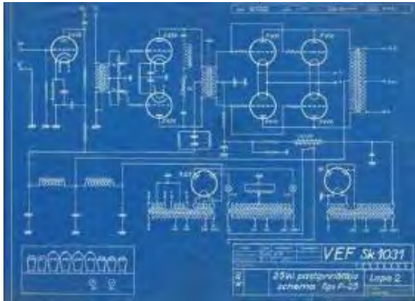
25 W pastiprinātājs
