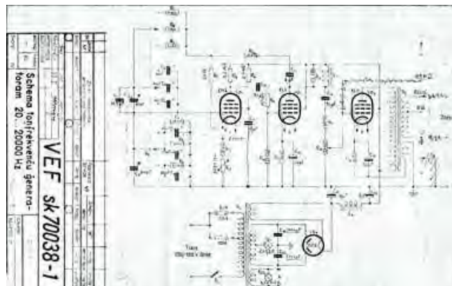
Tonfrequenču ģenerators
