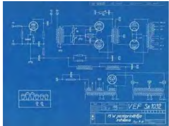
15 W pastiprinātājs
