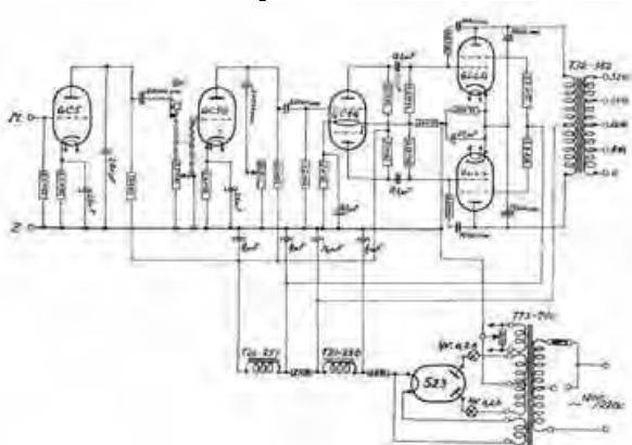
25 W pastiprinātājs
