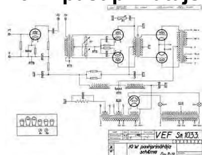
10 W pastiprinātājs
